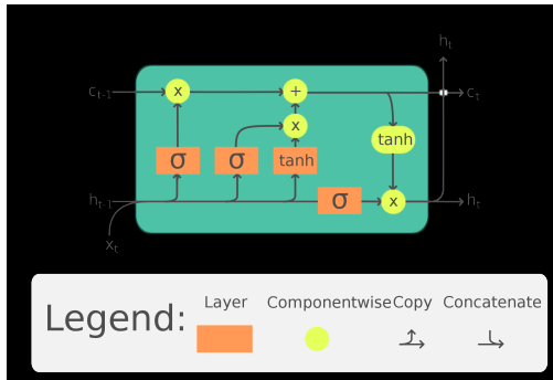
Abb. 2: Eine LSTM-Zelle [5] .
